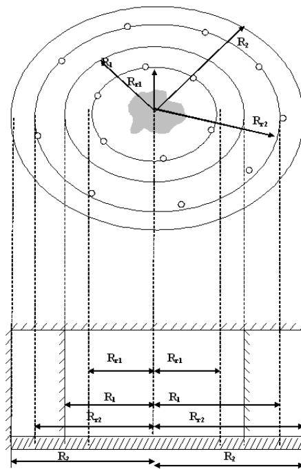
Рис. 1. Расположение батареи скважин вертикального дренажа в плане.
