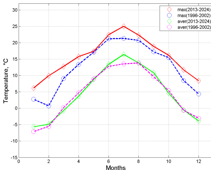
1-rasm. 1996-2002-yillarda oʻlchangan va 2013-2024-yillarda oʻlchangan temperaturalarning farqi
