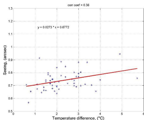
2-rasm. Maydanak observatoriyasida tun davomida temperatura o'zgarishining mavsumiy statistikasi (chap grafik) va uning tasvir sifatiga ta'siri (o'ng grafik)
